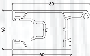
PB 108 SLIDING DOOR SASH (80*40)
