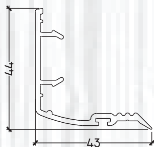
PB 112 SLIDING DOOR SASH INTERLOCK (44*43)
