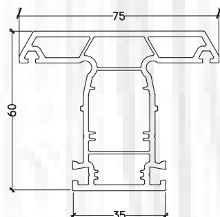
PB 208 CASEMENT T-MULLION
