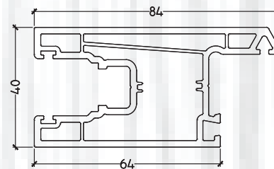
PB 109 SLIDING DOOR SASH (84*40)
